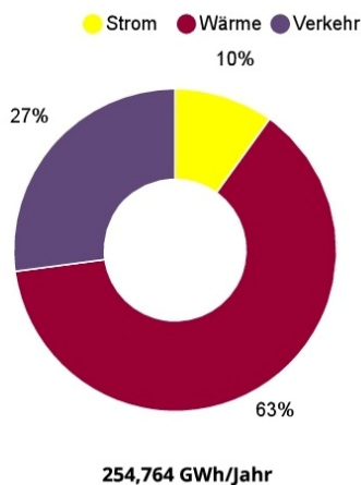
Endenergieverbrauch gesamt 2014
